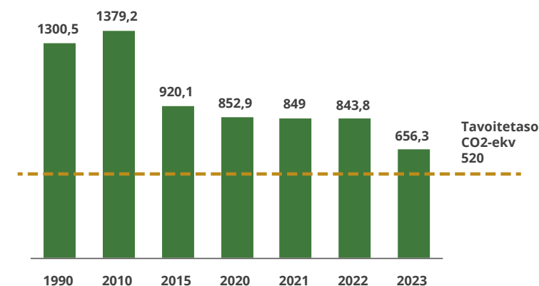
Hiilidioksidipäästöjen kehitys Tampereella ml. teollisuuden päästöt, kt CO 2 -ekv
